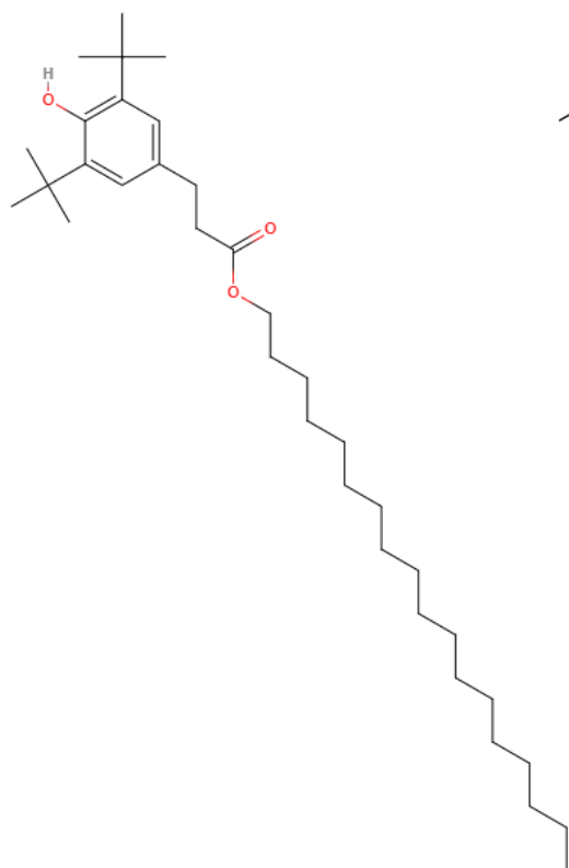
Irganox 1076
