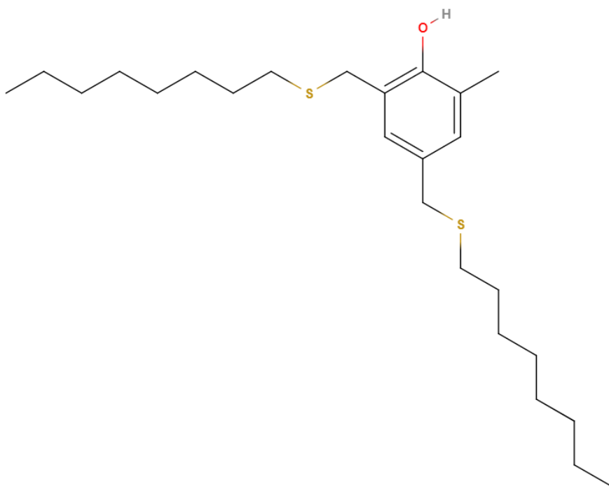
Irganox 1520
