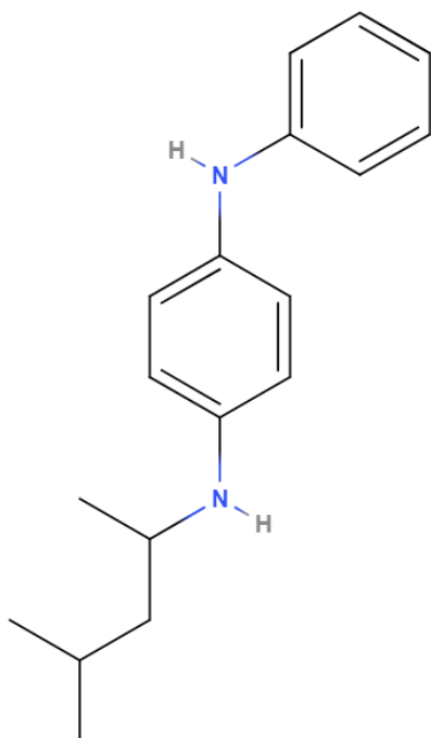
6PPD
