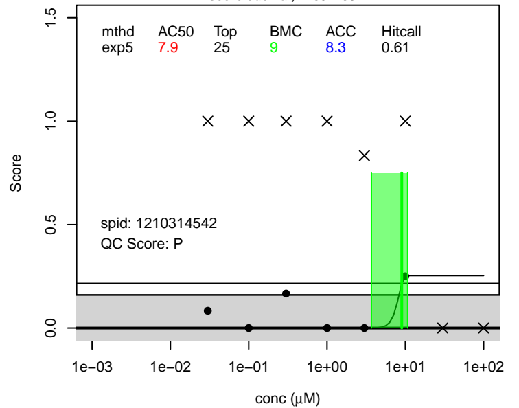
6:3 FTCA score.edema ; 27854-30-4
