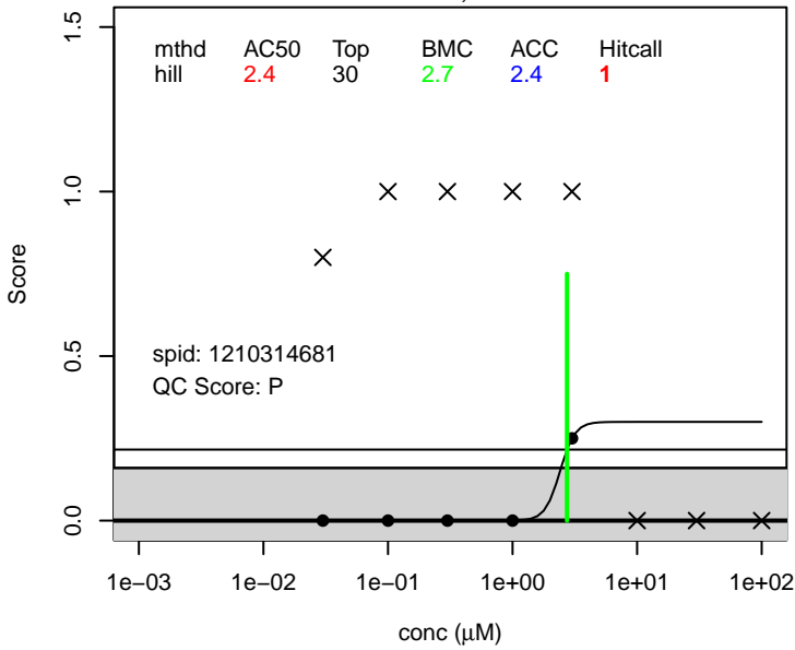
PFUnDA score.edema ; 2058-94-8
