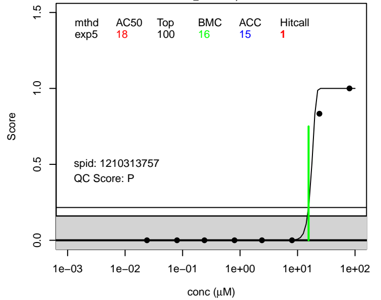
PFHpS score.edema ; 375-92-8
