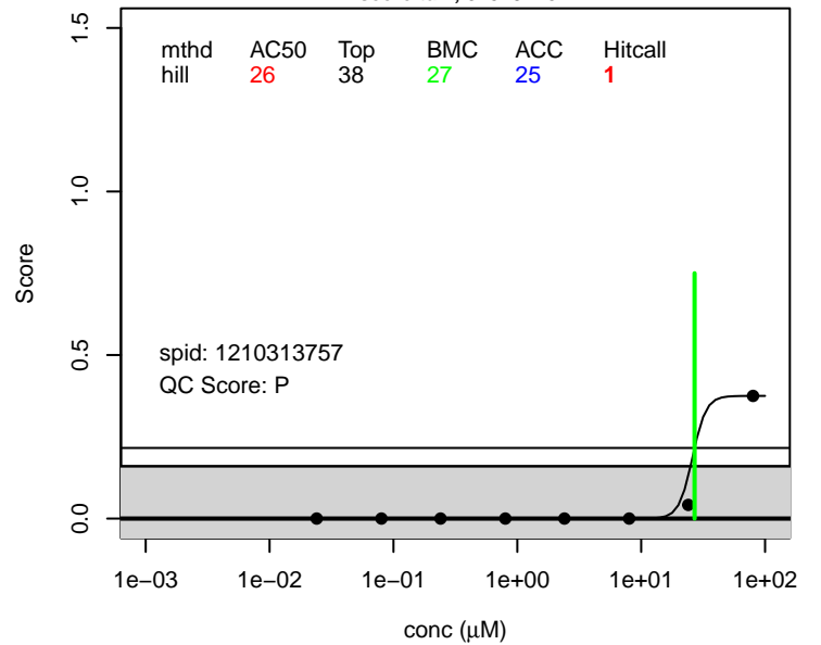
PFHpS score.tail ; 375-92-8
