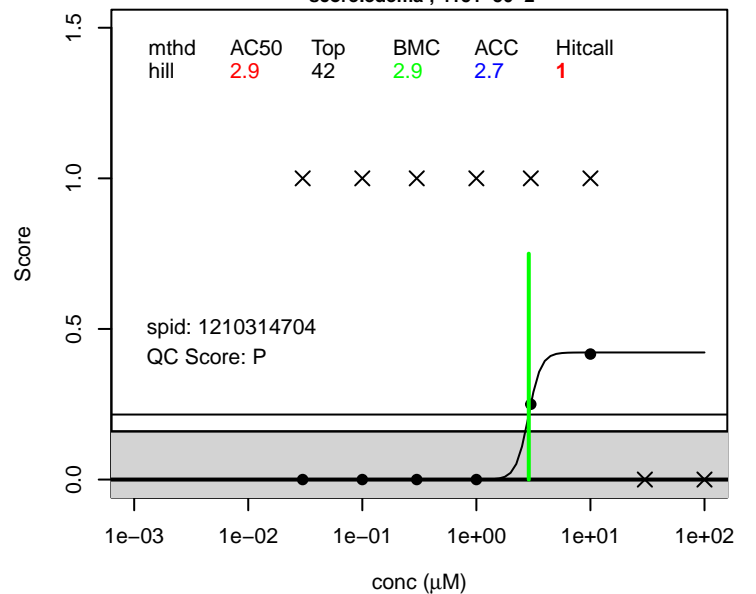
NEtFOSA score.edema ; 4151-50-2
