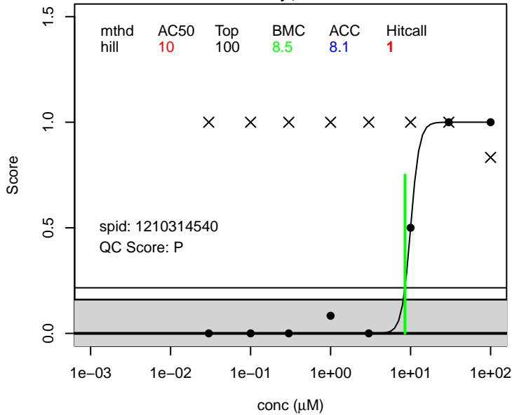
6:3 FTCA score.general ; 27854-30-4
