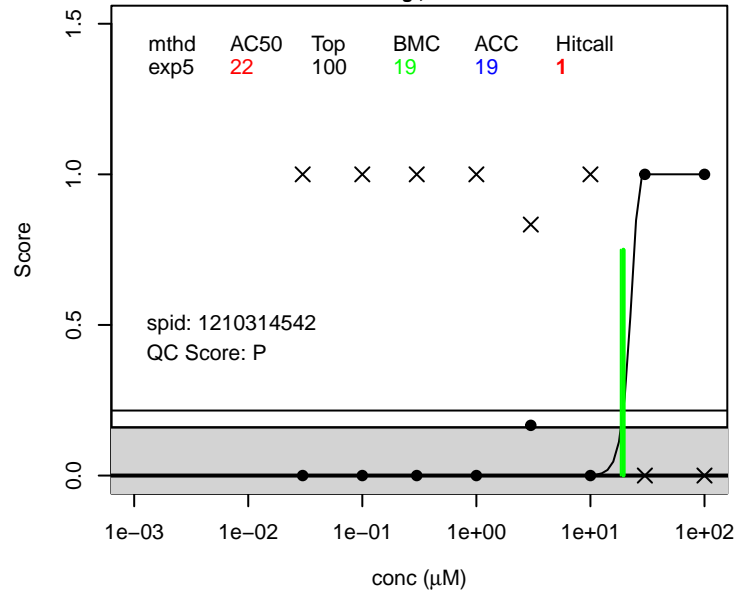
6:3 FTCA score.edema ; 27854-30-4
