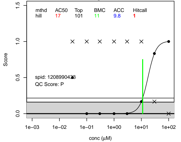
H-PFUnA score.edema ; 1765-48-6
