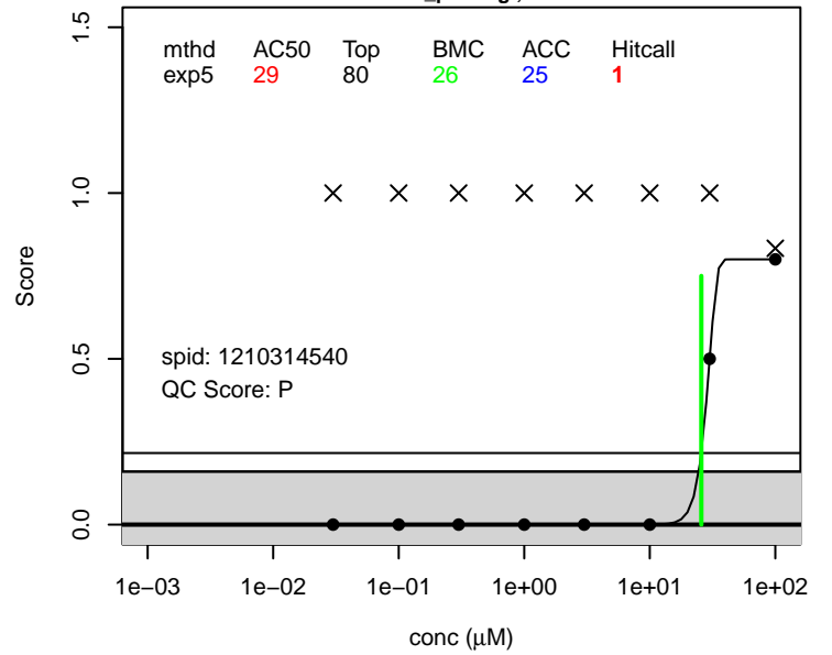
6:3 FTCA score.living ; 27854-30-4
