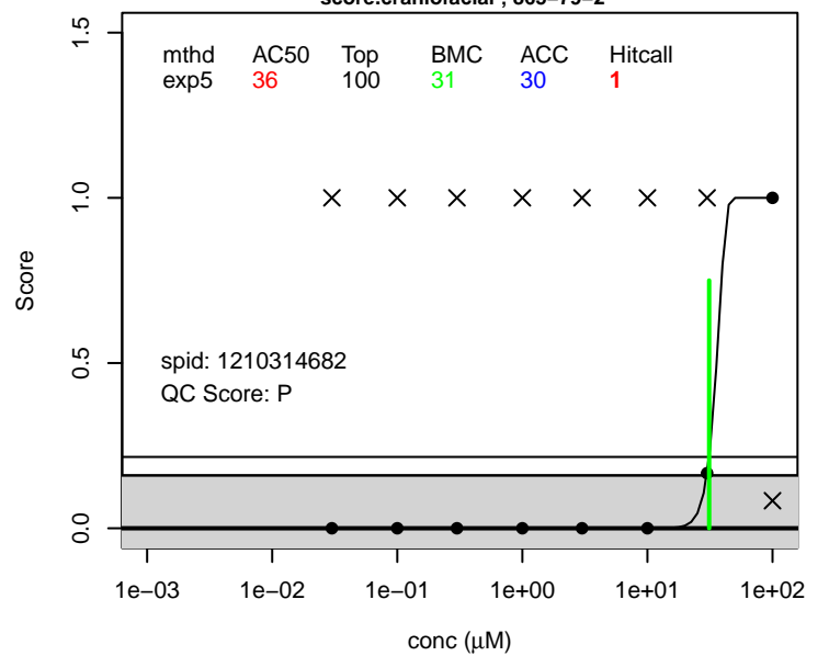
CI-PFNA score.craniofacial ; 865-79-2
