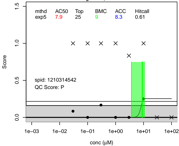
6:3 FTCA score.general ; 27854-30-4
