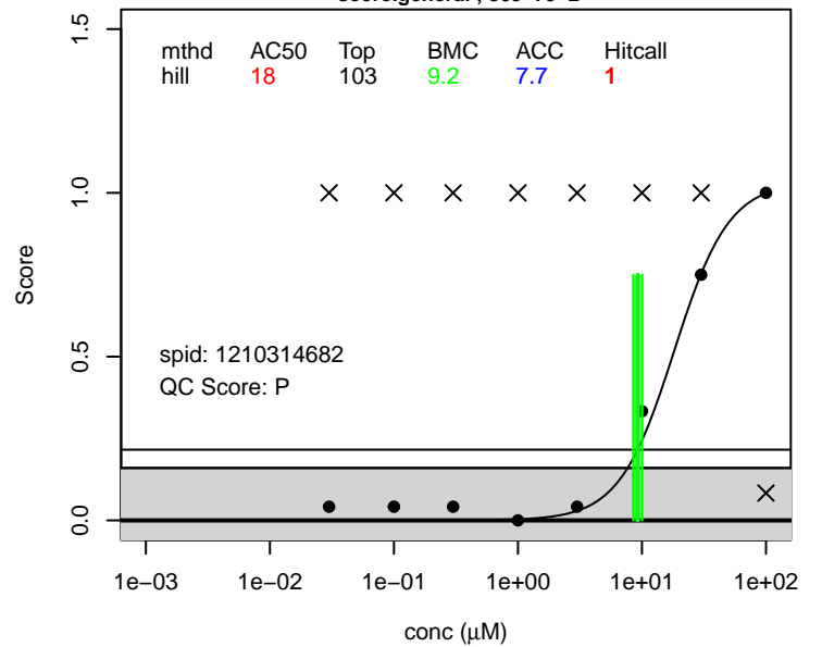
CI-PFNA score.craniofacial ; 865-79-2
