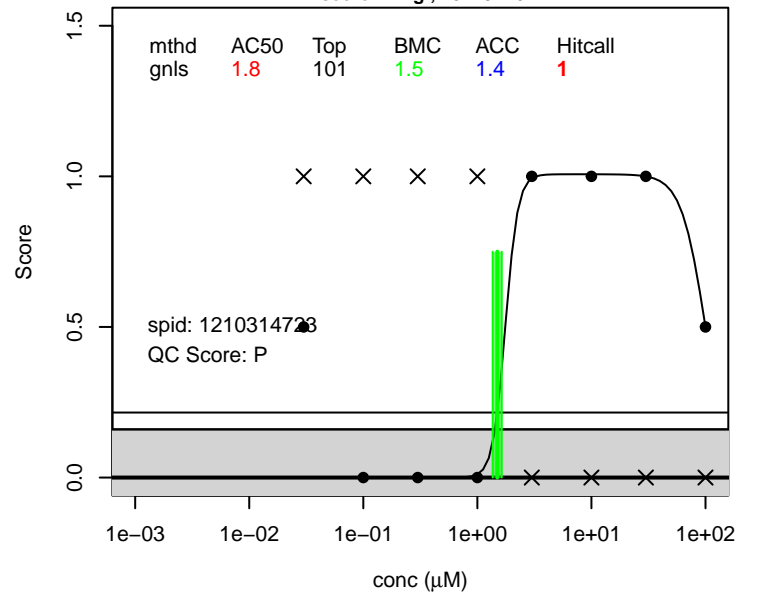
PFOSA score.living ; 754-91-6
