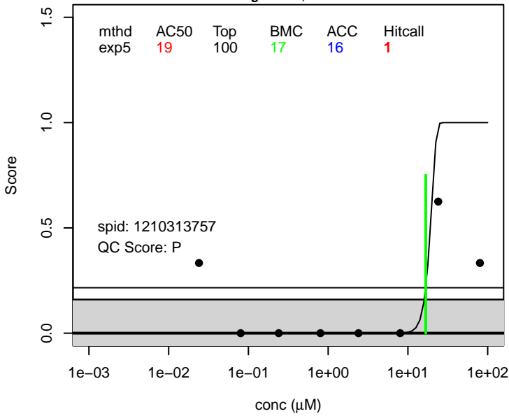
PFHpS score.craniofacial ; 375-92-8
