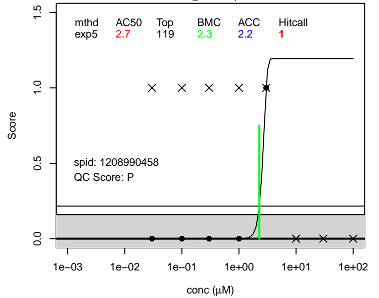
Perfluoropinacol score.edema ; 918-21-8
